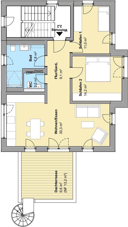
1. Obergeschoss
