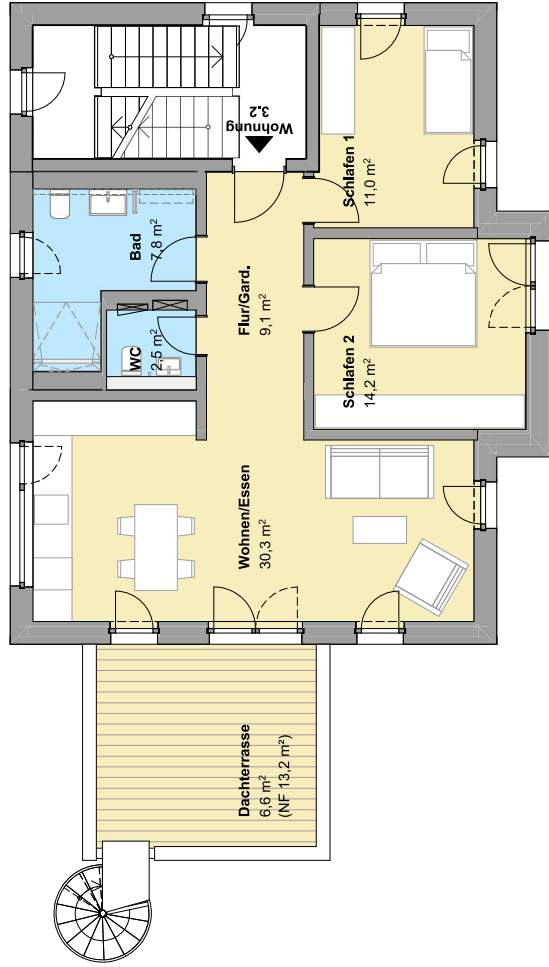
1. Obergeschoss
