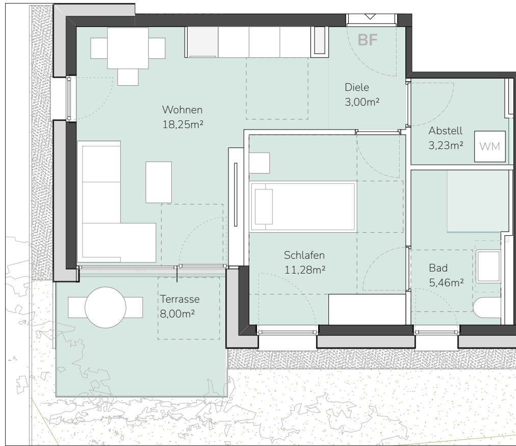
Haus A Grundriss Erdgeschoss - Wohnung E04
