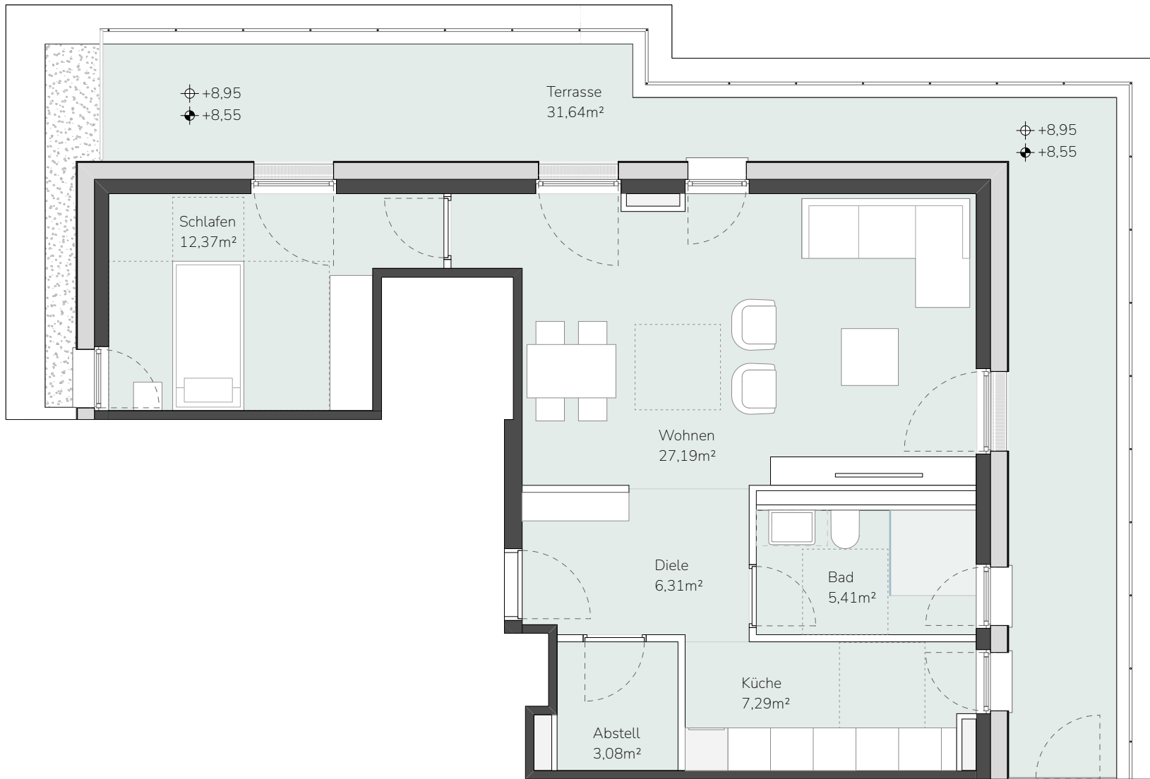
Haus B Grundriss Staffelgeschoss - Wohnung E31
