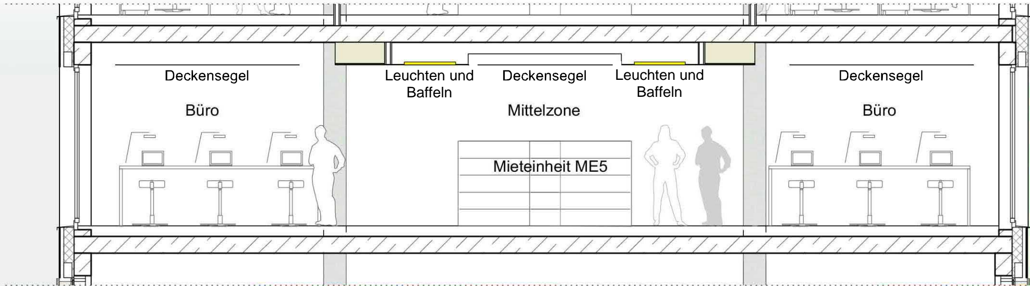
Schemaschnitt Büro
